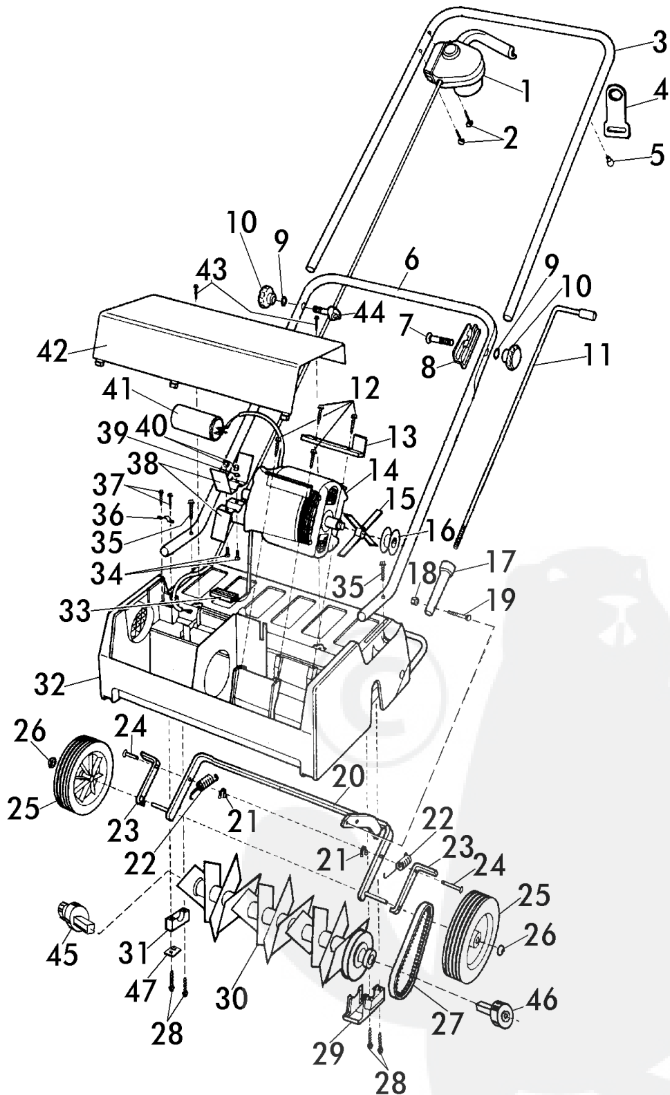
ELEKTRO - VERTIKUTIERER 35 Art. 75094 (ab Bj. 1990)
