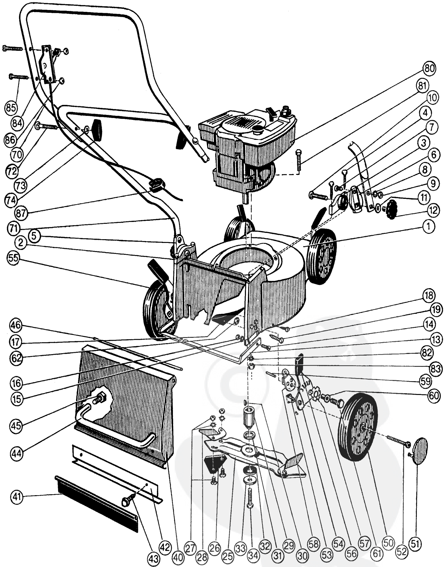
Roto - KING 46 N Typ 1122
