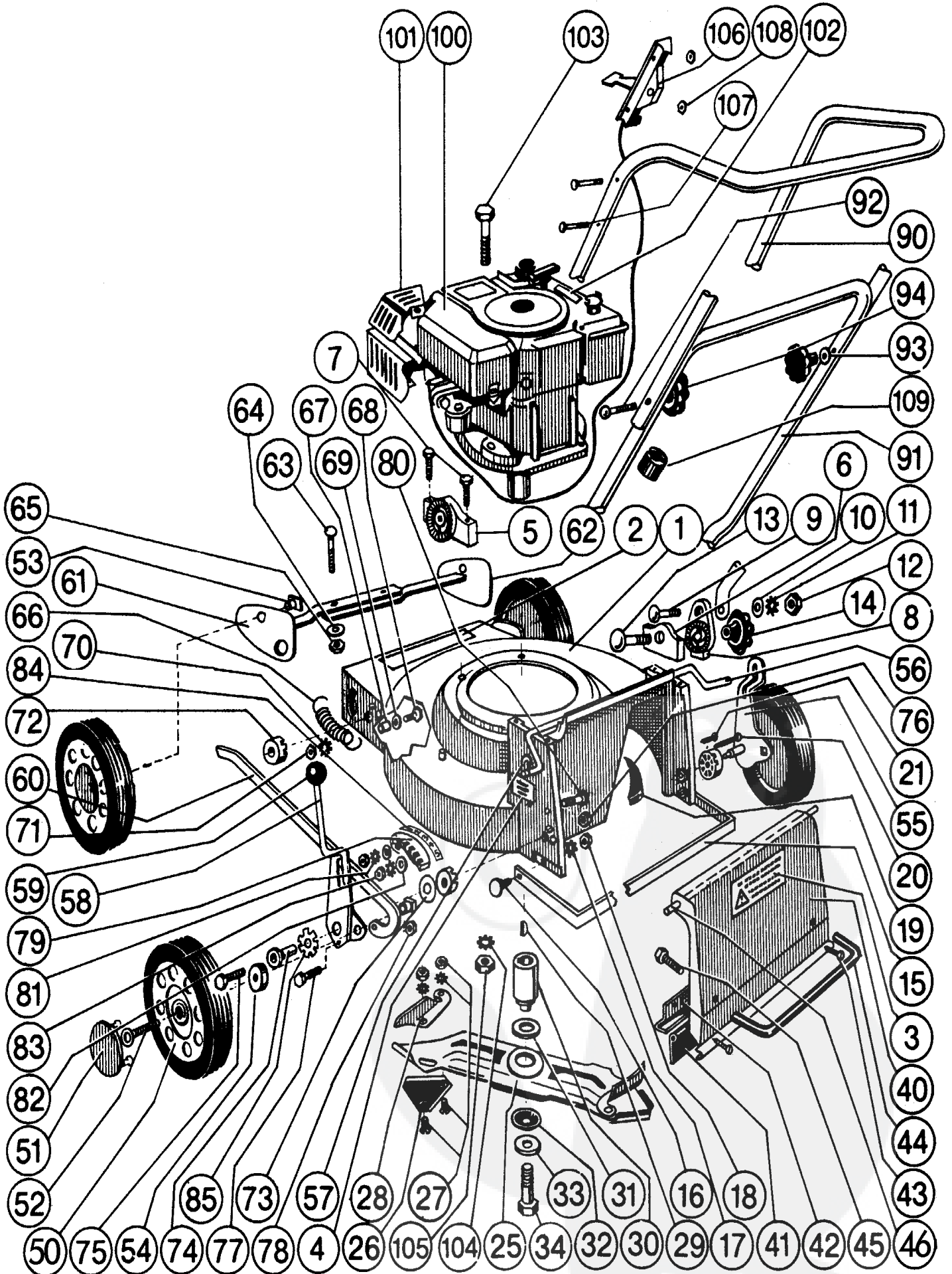
ROTO - PRINZ 40 TYP 1012 + 71012
